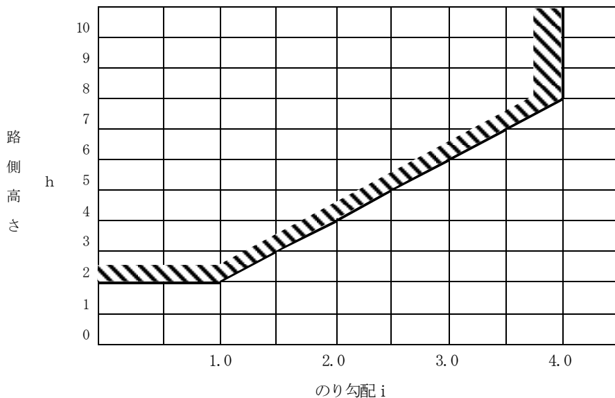
h : 路側高さ (m) i : のり勾配 (割)
