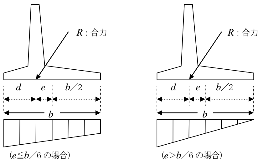
擁壁底面の地盤反力
