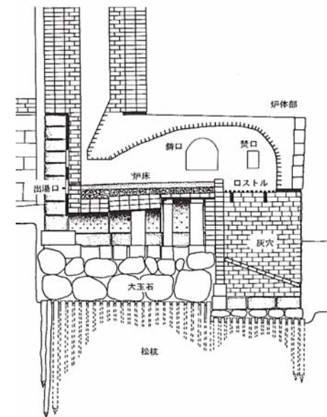
反射炉の基礎構造（断面図）
