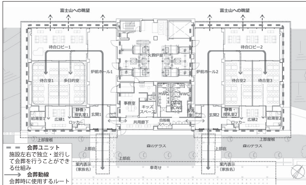
▲1階平面図
