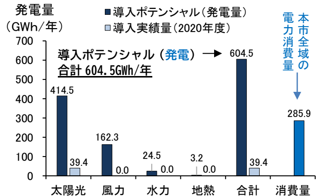
導入ポテンシャル（発電）と導入実績量（2020年度） 注）導入実績量は固定価格買取制度（FIT）のデータ。 【資料：環境省・自治体再エネ情報カルテより作成】
